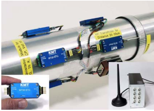
旋轉體用微型量測設備
